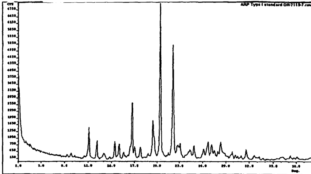
Figura 1. Difractograma de rayos X de aripiprazol de tipo I
