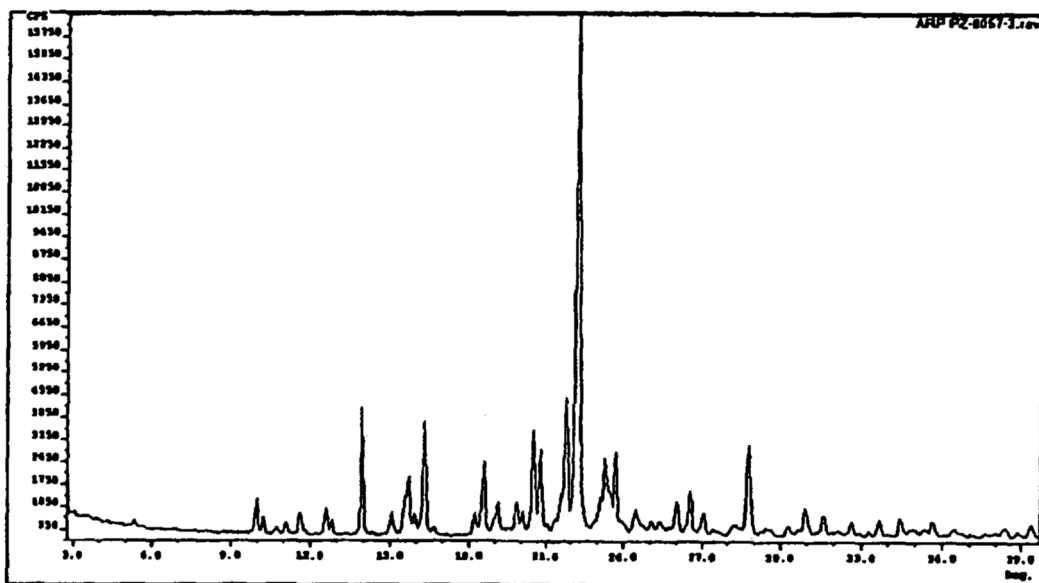
Figura 2. Difractograma de rayos X de aripiprazol de tipo II
