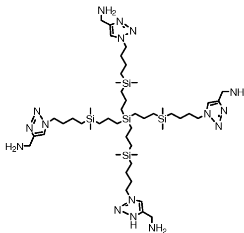
ck\text{-G}_1\text{-[Si(CH}_2)_4(\text{N}_3\text{C}_2\text{H})\text{CH}_2\text{NH}_2]_4
