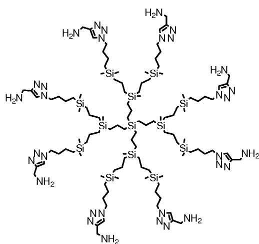
ck\text{-G}_2\text{-[Si(CH}_2)_4(\text{N}_3\text{C}_2\text{H})\text{CH}_2\text{NH}_2]_8
