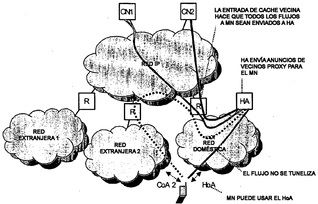
FIGURA 3. DISTRIBUCIÓN DE PAQUETES A NODO MÓVIL EN RED DOMÉSTICA
