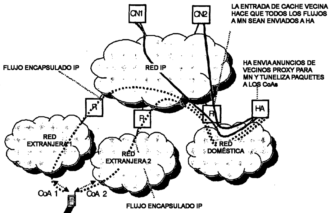
FIGURA 1: USO DE ENLACES MÚLTIPLES EN REDES EXTRANJERAS
