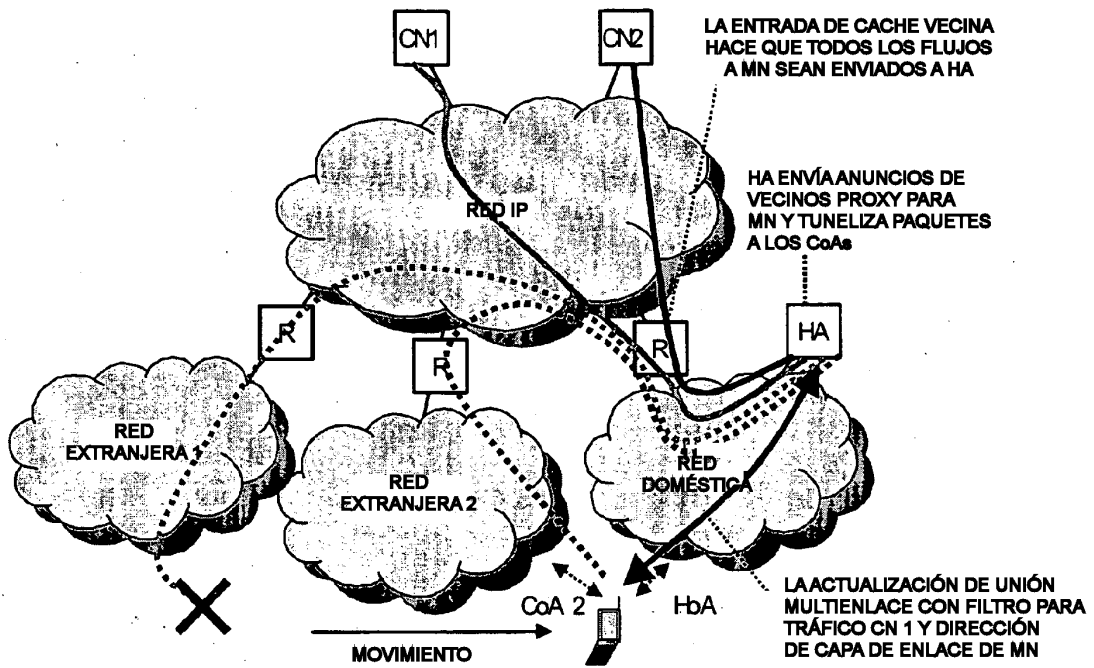
FIGURA 2: REGISTRAR INTERFACE DE ENLACE DOMÉSTICO CON AGENTE DOMÉSTICO
