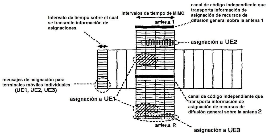
Transmisión de información de asignación de recursos de difusión general a través de un canal de código independiente
