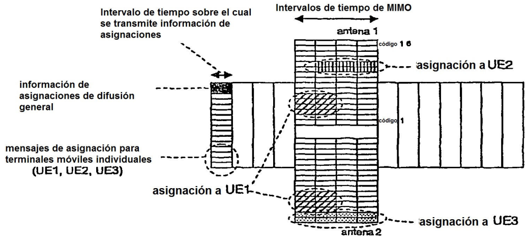
Ejemplo de información de asignación de códigos de difusión general en el TDD UTRA
