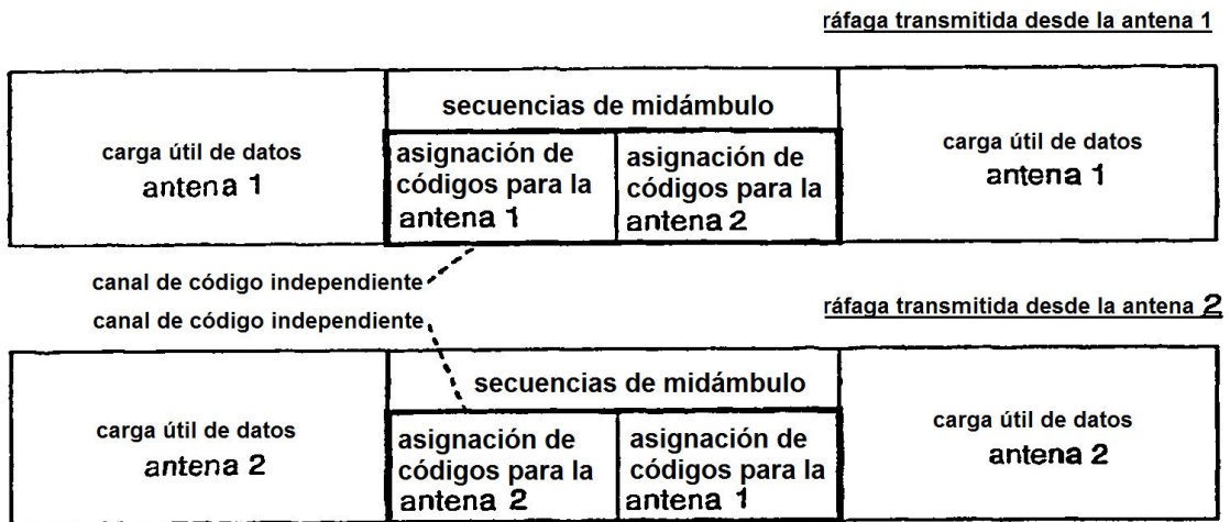
Transmisión de difusión general de información de asignación de códigos en la parte del midámbulo de la ráfaga
