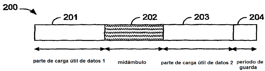
Configuración de los intervalos de tiempo TDD UTRA
