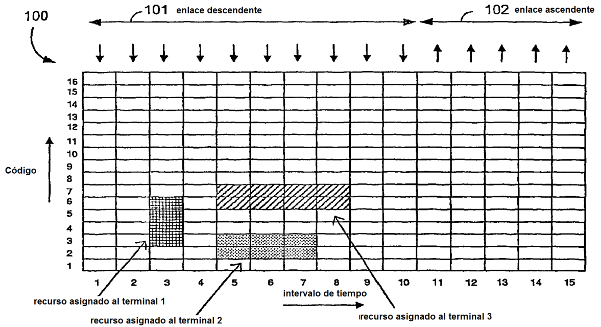
Trama de radiocomunicaciones TDD típica
