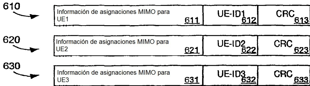
Estructura de HS-SCCH para difundir de forma general implícitamente información de asignaciones
