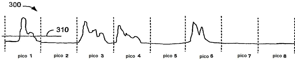
Señal de ejemplo en la salida de un detector de midámbulos TDD
