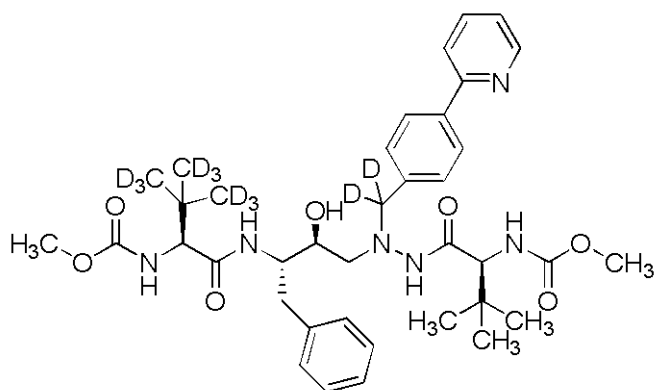
Compuesto 111
