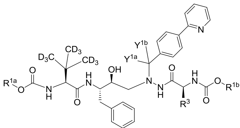
(Ib)
