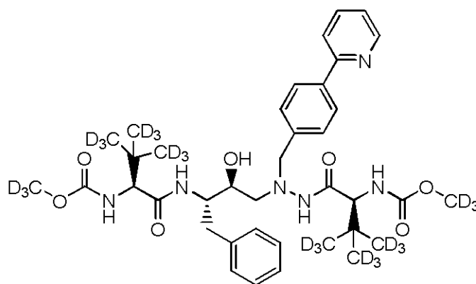
Compuesto 122
