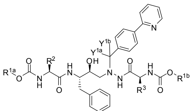
(Ia)
