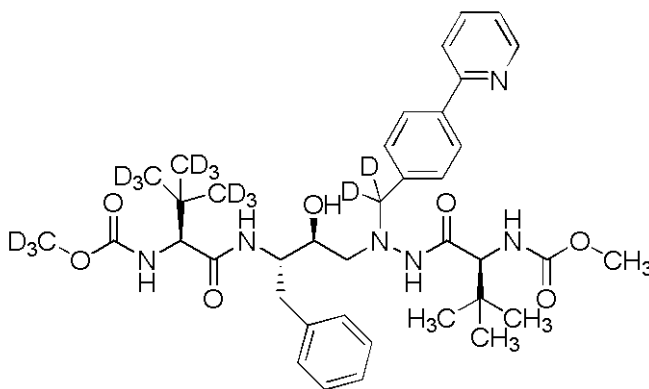
Compuesto 123
