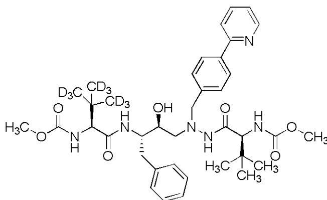
Compuesto 104
