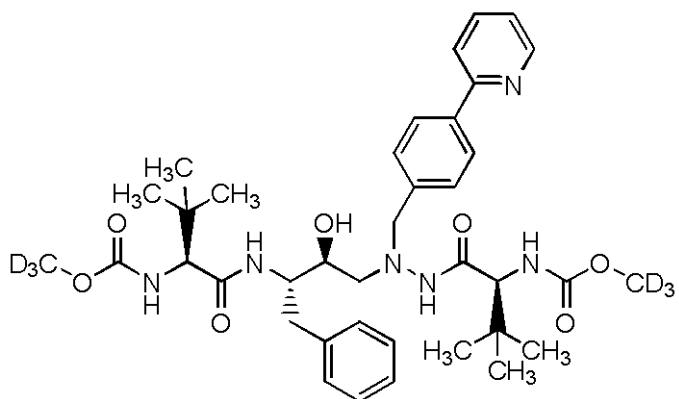
Compuesto 103
