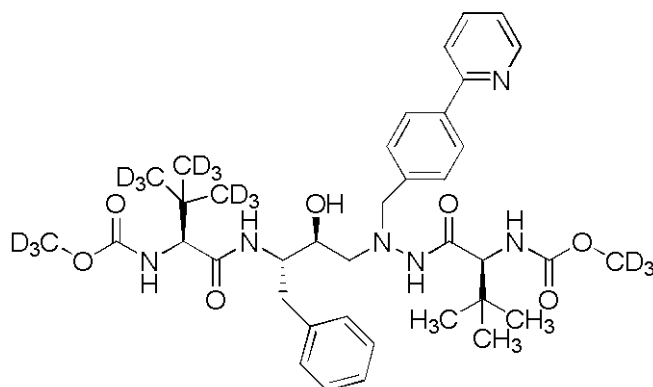
Compuesto 120
