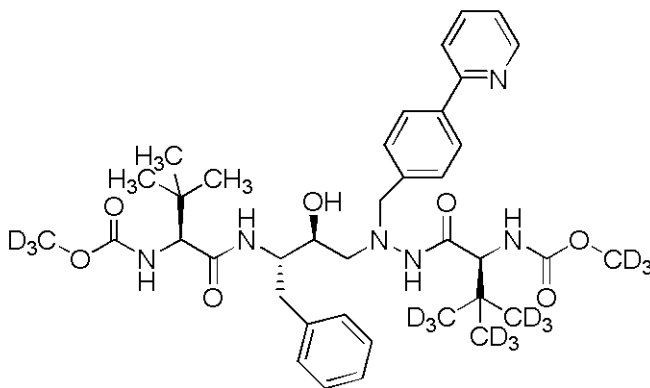
Compuesto 121
