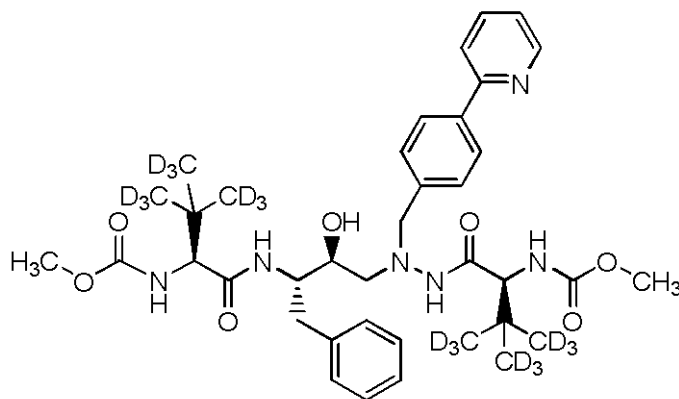
Compuesto 106
