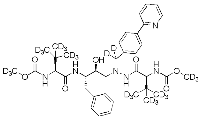
Compuesto 131
