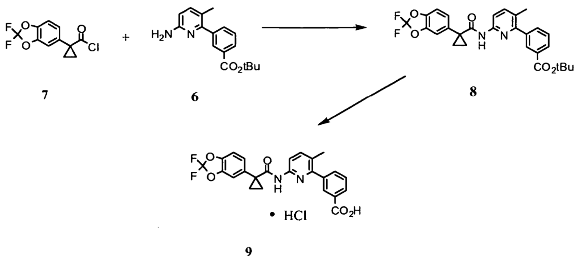
Esquema 3. Formación de una sal de ácido de ácido 3-(6-(1-(2,2-difluorobenzo[d][1,3]dioxol-5-il)ciclopropanocarboxamido)-3-metilpiridin-2-il)benzoico
