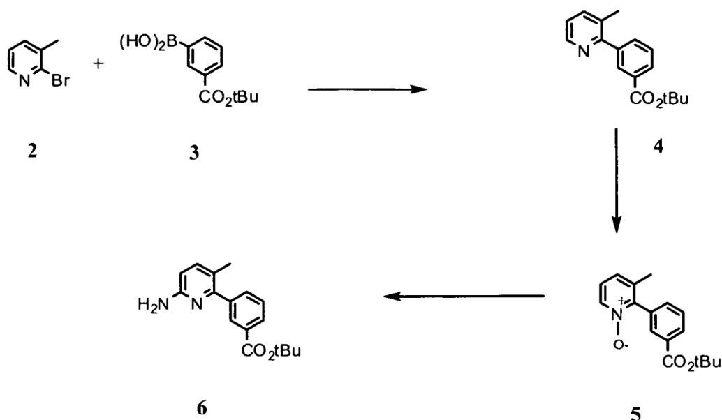
Esquema 2. Síntesis del resto amina
