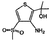
4-metanosulfonil-tiofeno (2,26)
