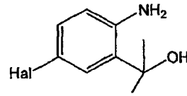
alcohol 4-bromobencílico (3,82)
