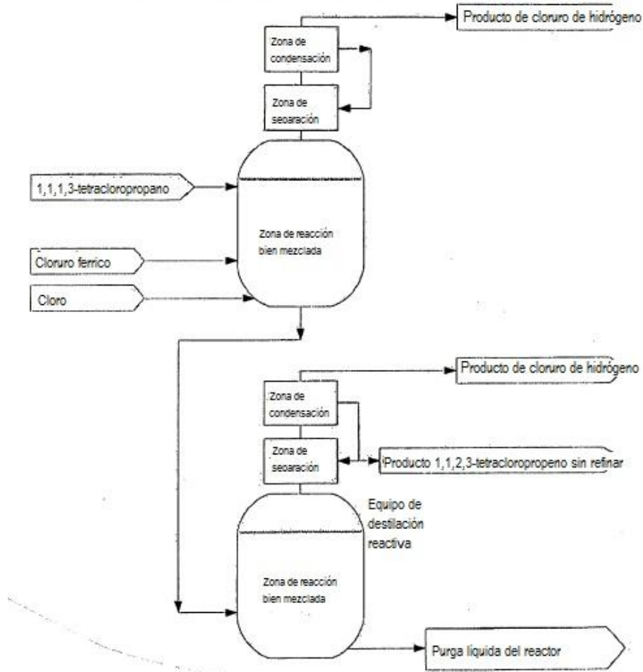
Figura 3. Un proceso de la invención para hacer 1,1,2,3-tetracloropropano
