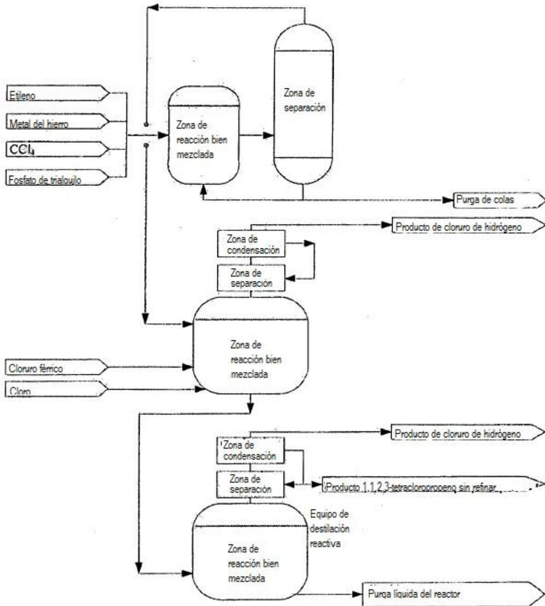
Figura 4. Un proceso de la invención para hacer 1,1,2,3-tetracloropropeno
