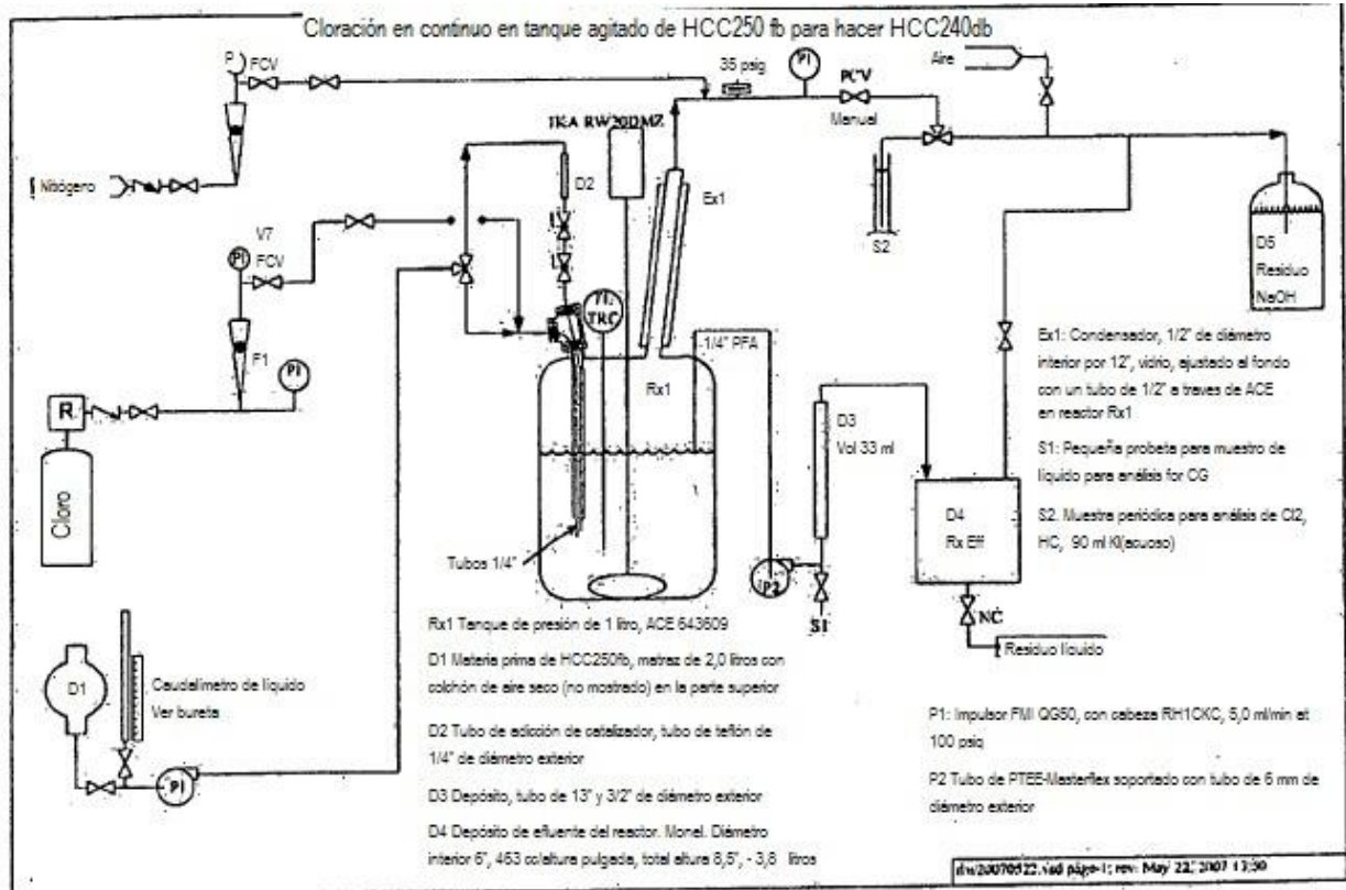
Figura 6. Equipo de laboratorio para la reacción en continuo de HCC240db
