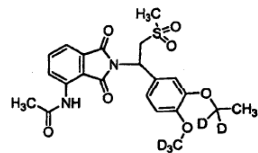
Compuesto 108
