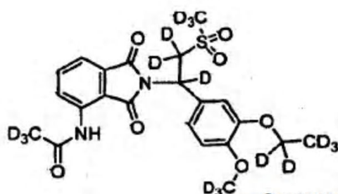
Compuesto 101,
