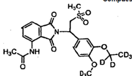
Compuesto 107,
