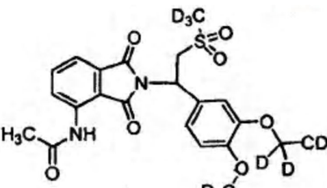
Compuesto 106,
