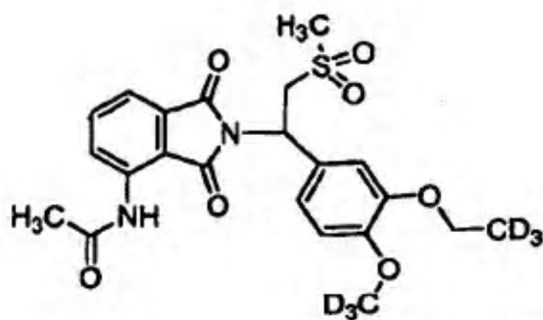
Compuesto 109,
