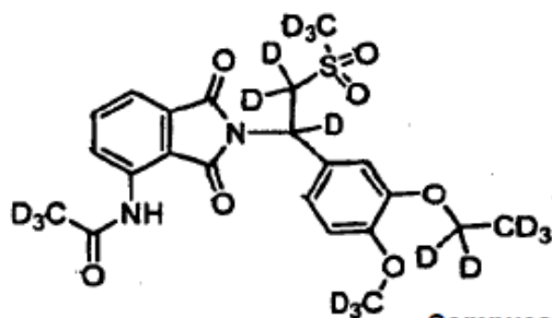
Compuesto 101,
