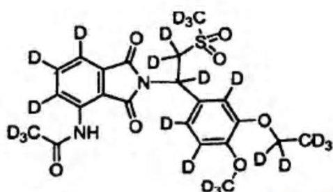
Compuesto 100,
