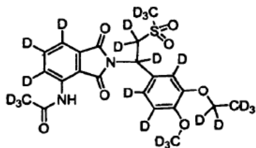
Compuesto 100,
