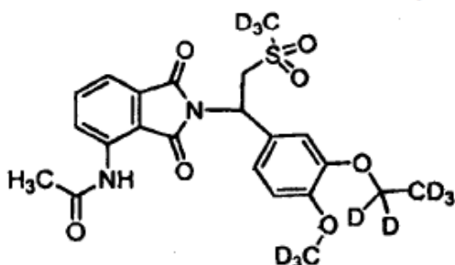
Compuesto 106,
