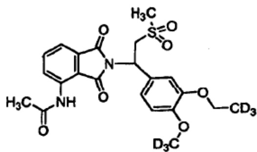
Compuesto 109,
