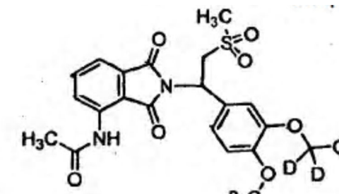
Compuesto 107,
