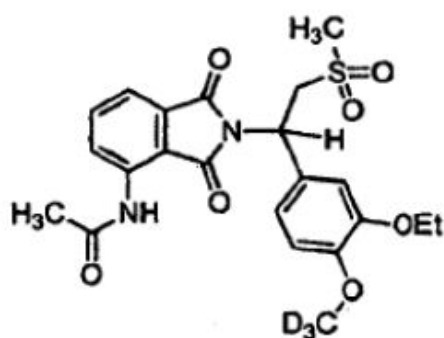
Compuesto 114,
