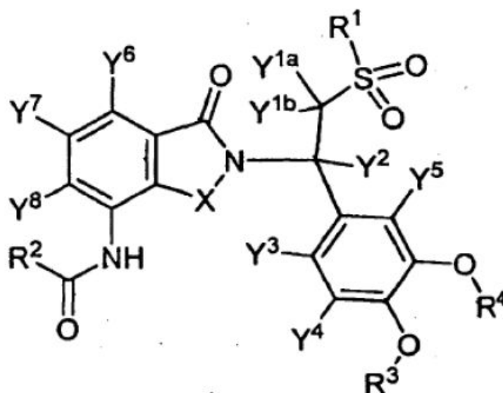
Fórmula I
