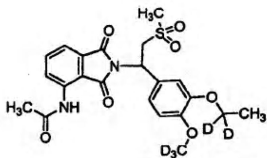
Compuesto 108
