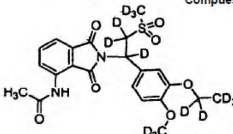
Compuesto 104,
