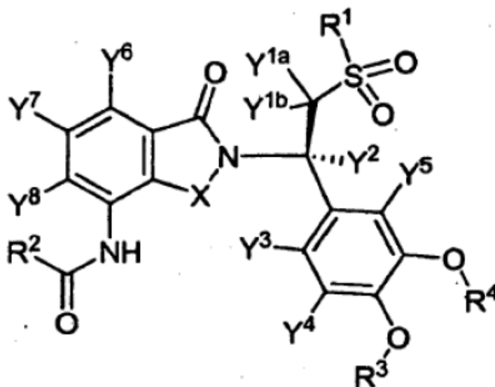
Fórmula Ib
