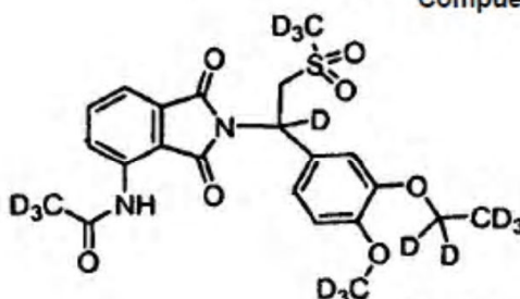
Compuesto 102,
