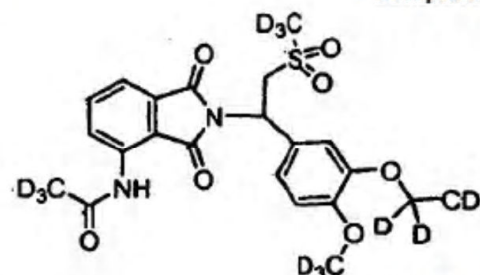
Compuesto 103,
