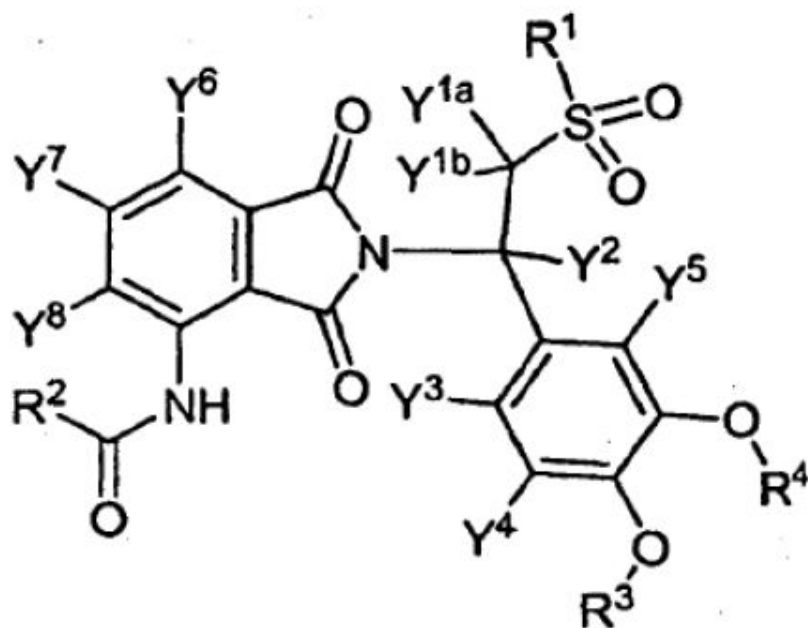
Fórmula II
