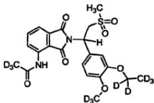
Compuesto 115 y
