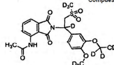
Compuesto 105,
