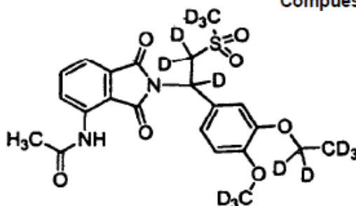
Compuesto 104,
