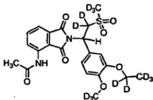
Compuesto 116,
