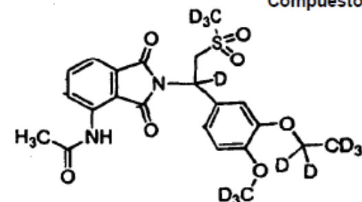
Compuesto 105,
