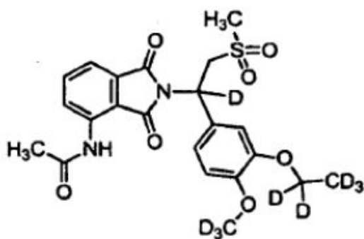
Compuesto 113,
