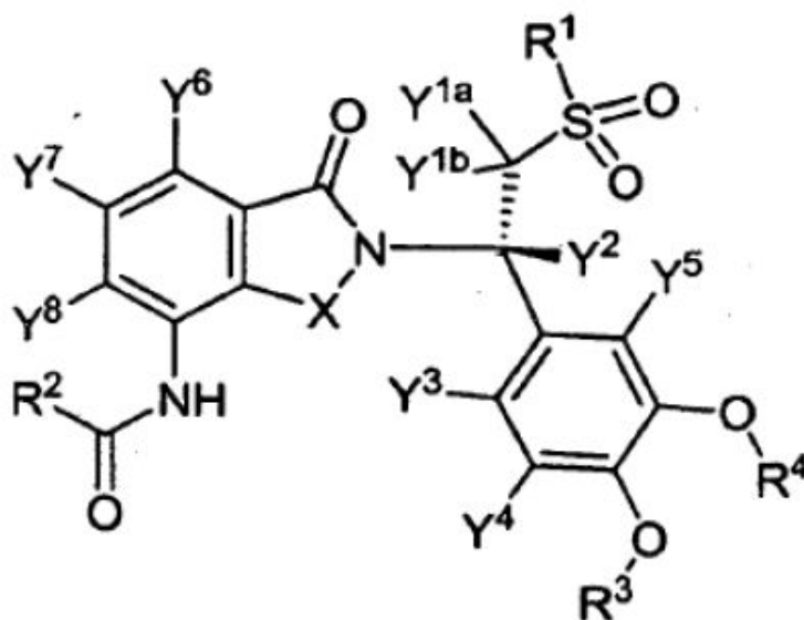
Fórmula Ia
