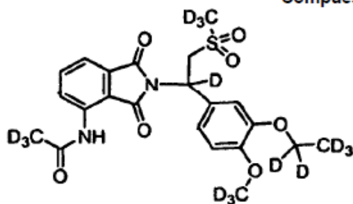
Compuesto 102,
