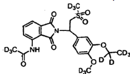
Compuesto 103,
