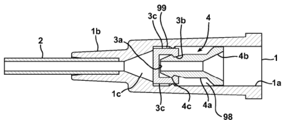
FIG. 2 Técnica Anterior
