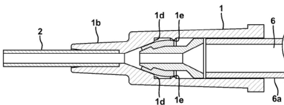
FIG. 3 Técnica Anterior
