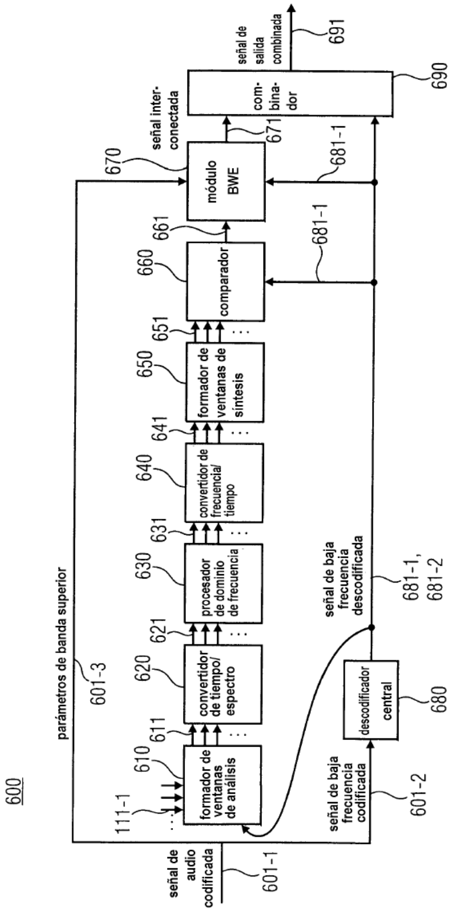
FIG 6 (LADO DEL DESCODIFICADOR)
