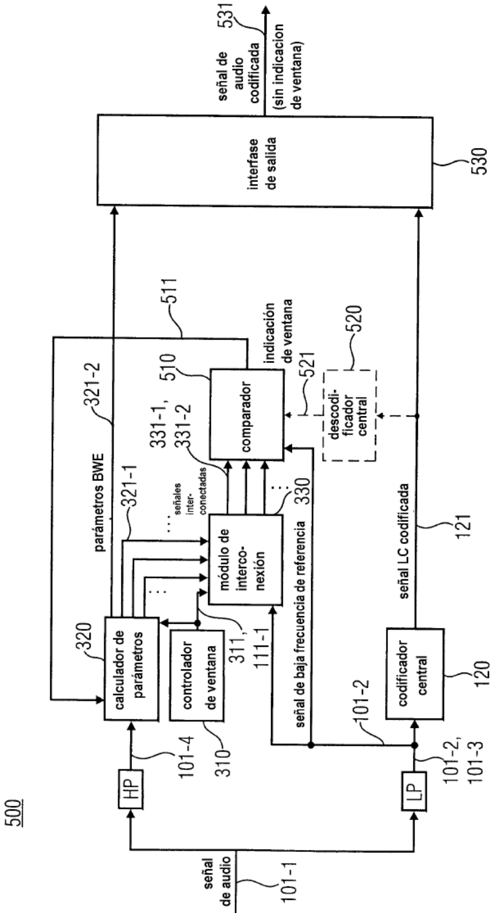
FIG 5 (LADO DEL CODIFICADOR)
