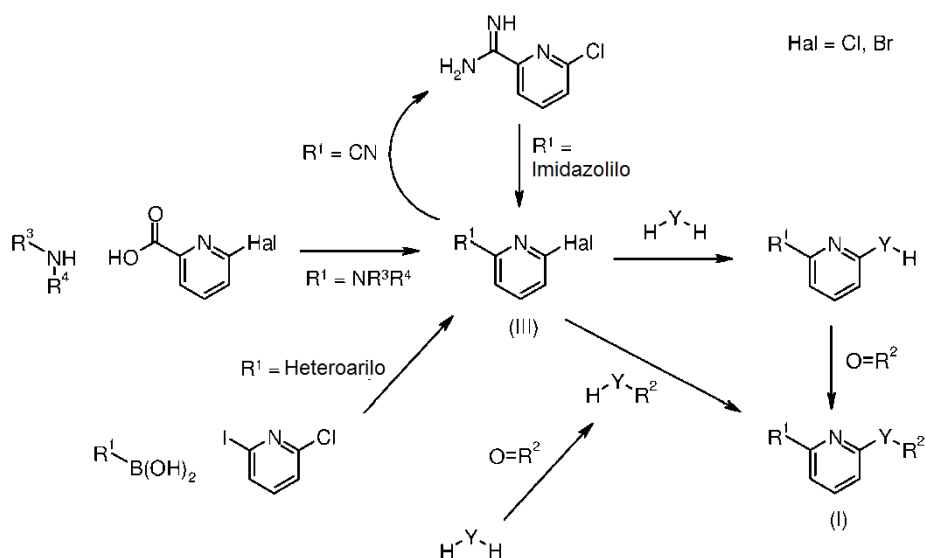
Esquema 1. Preparación de compuestos de fórmula (I) en donde X es un radical 2,6-piridilo de fórmula (A).
