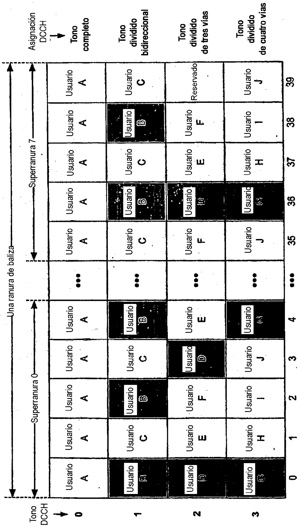
Segmento DCCH
