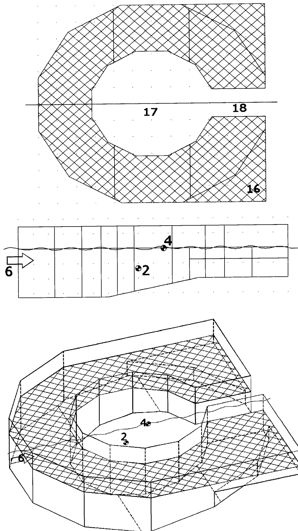
Figura 6 - Combinación de Variación de Calado y Flotador parcialmente sumergido en popa
