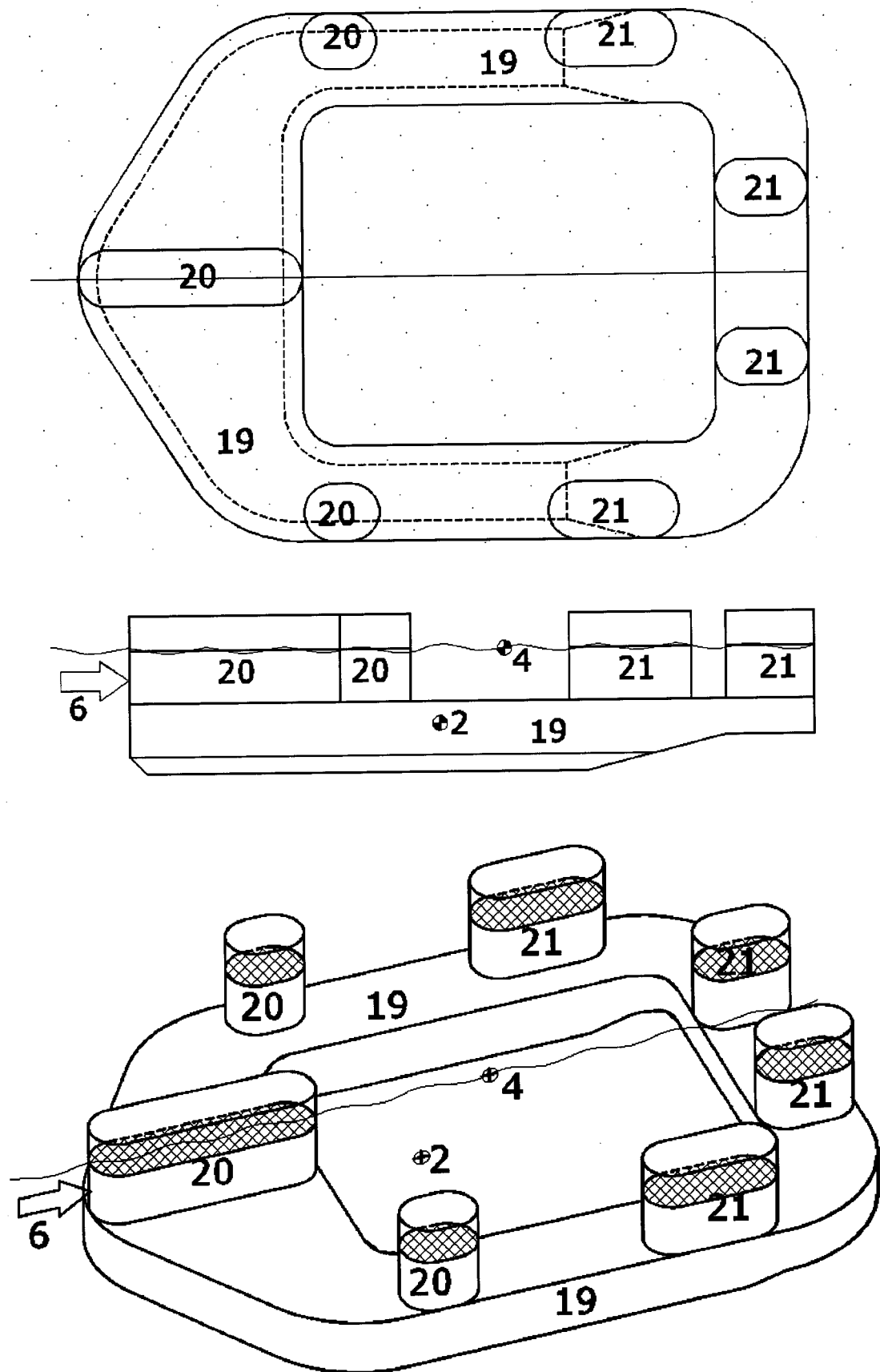
Figura 9 - Casco y columnas de forma arbitraria
