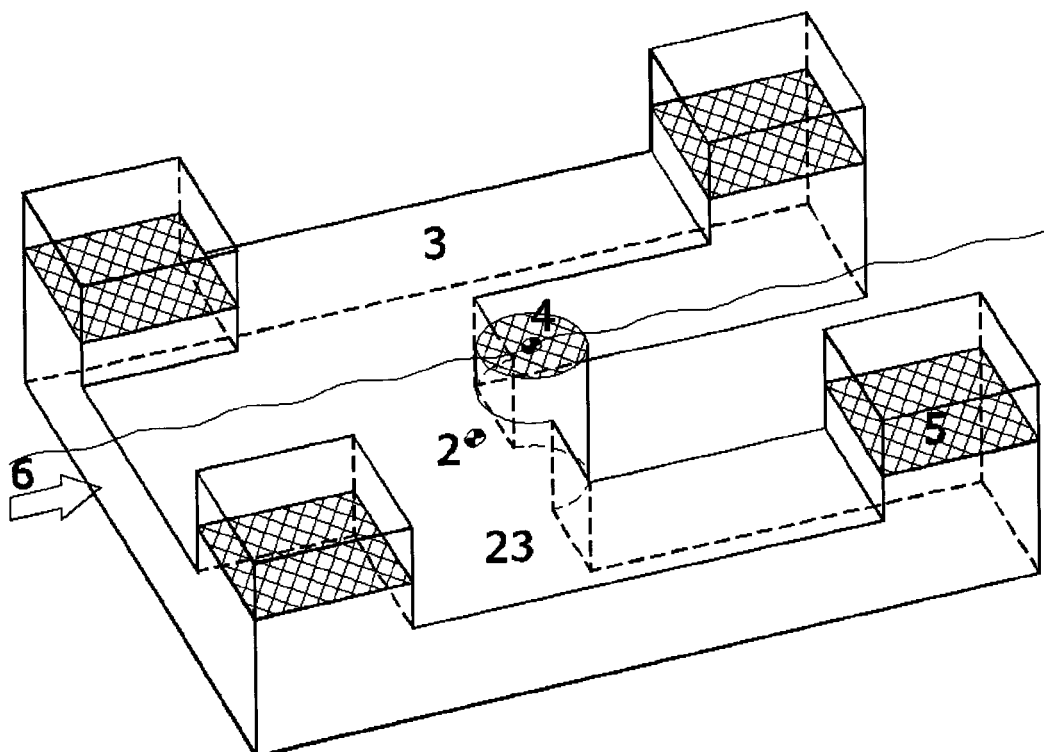
Figura 11 - Plataforma con columnas, adaptada para Aerogeneradores
