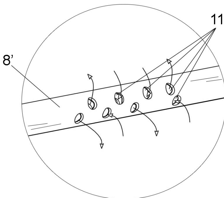
FIG. 4 DETALLE "A"
