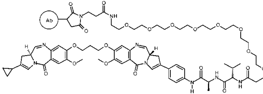
ConjA
