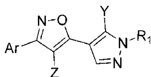
fórmula (I)
