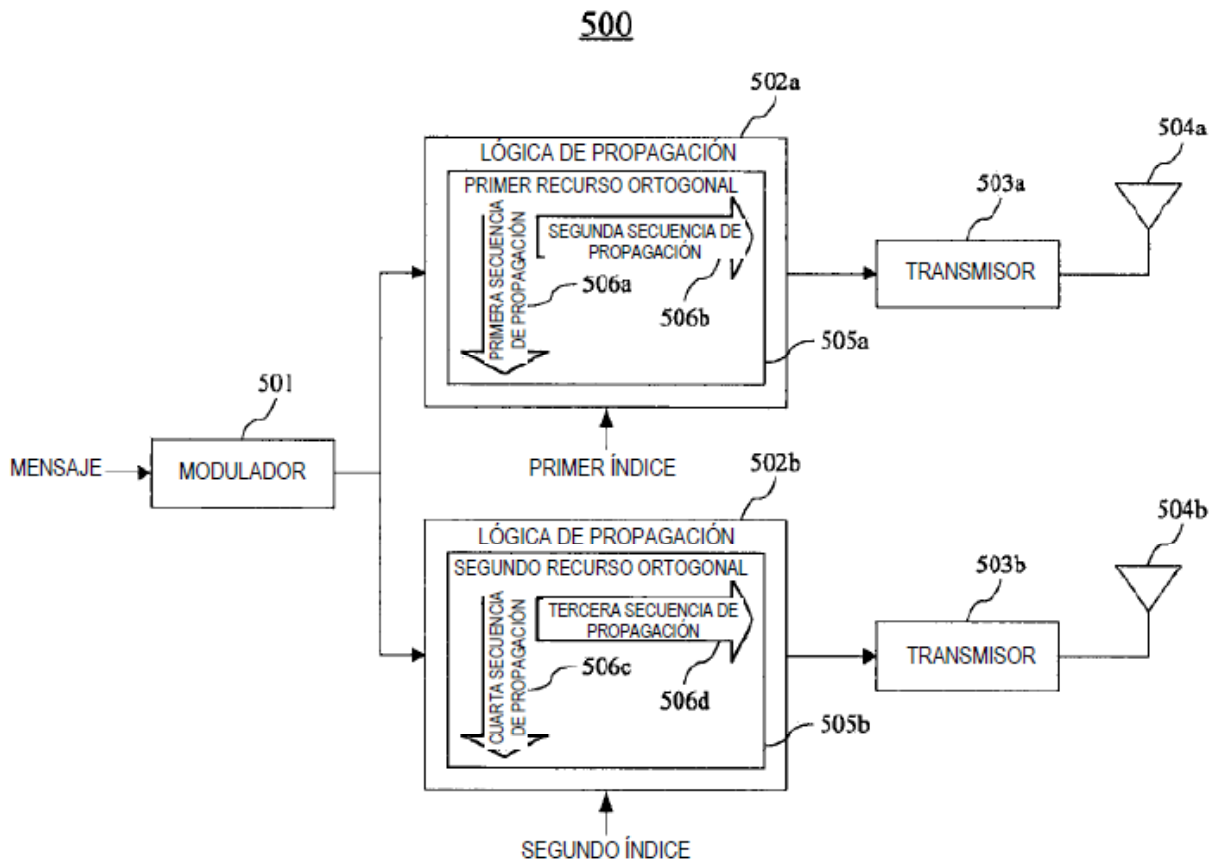
FIG. 5 (TÉCNICA ANTERIOR)
