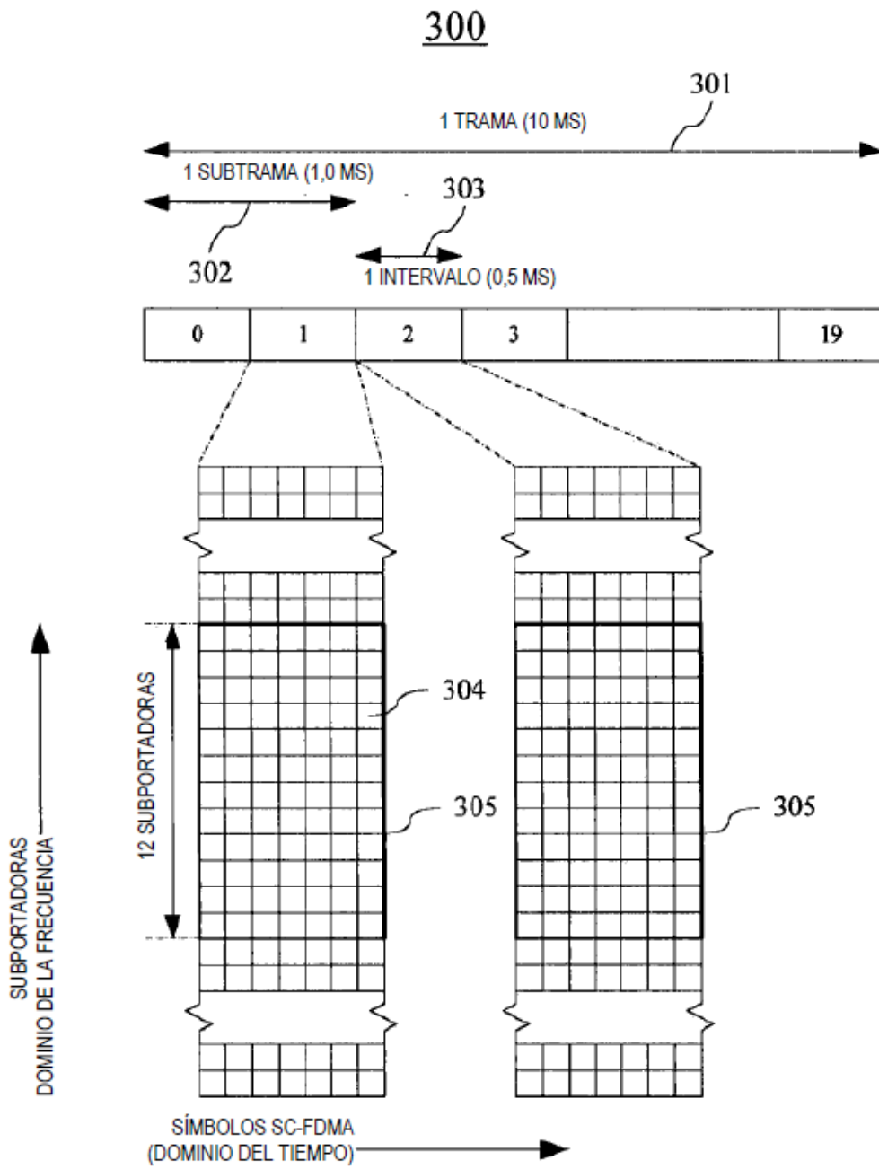
FIG. 3 (TÉCNICA ANTERIOR)
