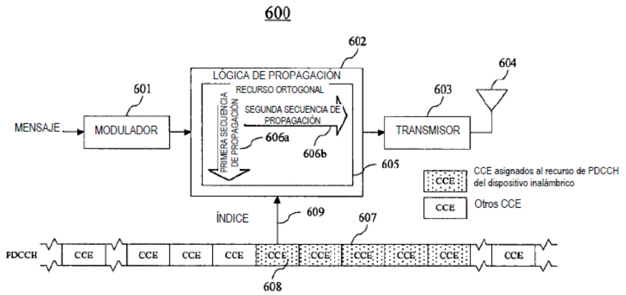
FIG. 6 (TÉCNICA ANTERIOR)
