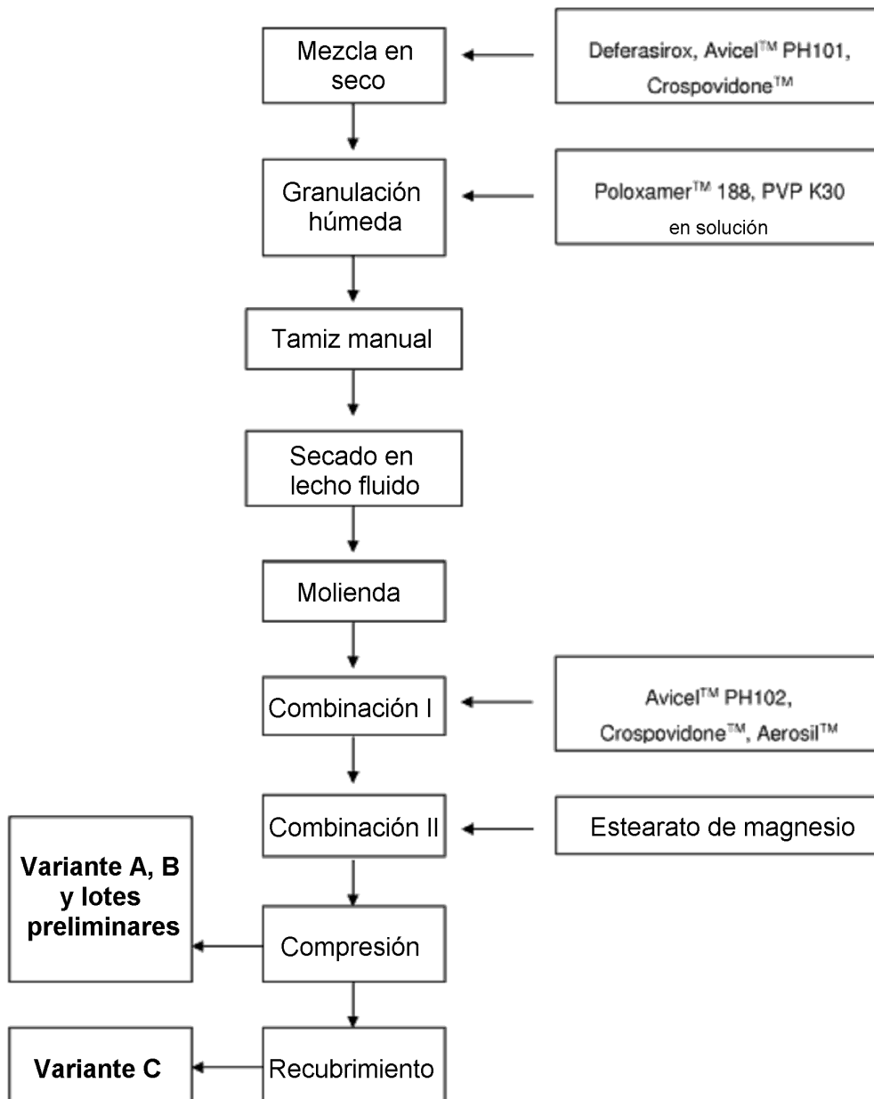
Figura 1: Proceso de producción de comprimidos de deferasirox recubiertos preparados mediante granulación húmeda
