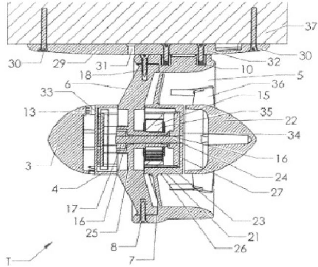
FIG. 3 VISTA DE LA SECCIÓN TRANSVERSAL
