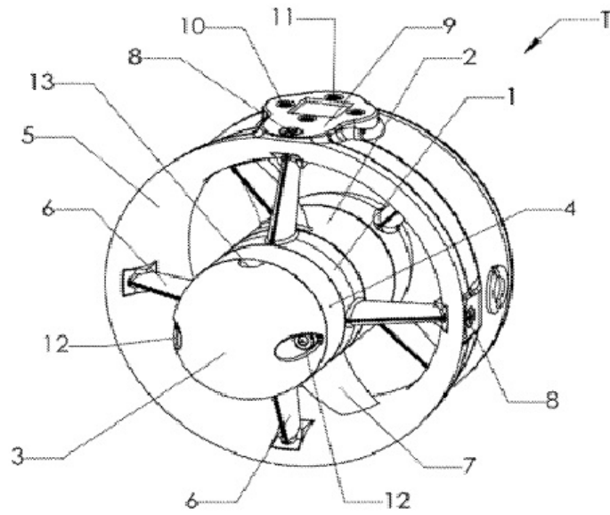
FIG. 1 VISTA ISOMÉTRICA
