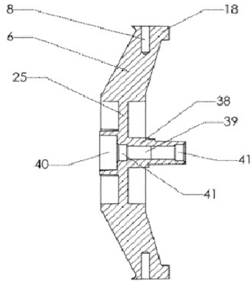
FIG. 4 VISTA DE LA SECCIÓN TRANSVERSAL DE LA BASE, BRAZOS DE LA BOQUILLA Y TUBO DE RODAMIENTO
