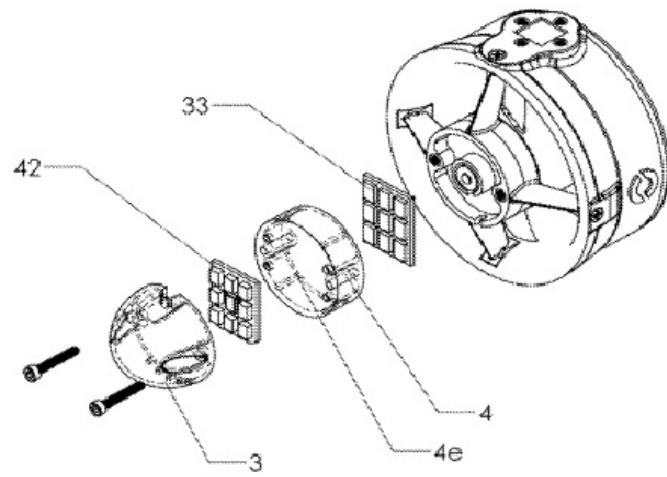
FIG. 5 VISTA EN DESPIECE ORDENADO CON LA UNIDAD ELECTRÓNICA Y EL LED DEL CONO DE OJIVA
