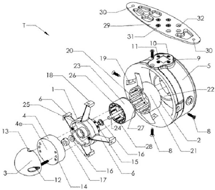
FIG. 2 VISTA EN DESPIECE ORDENADO
