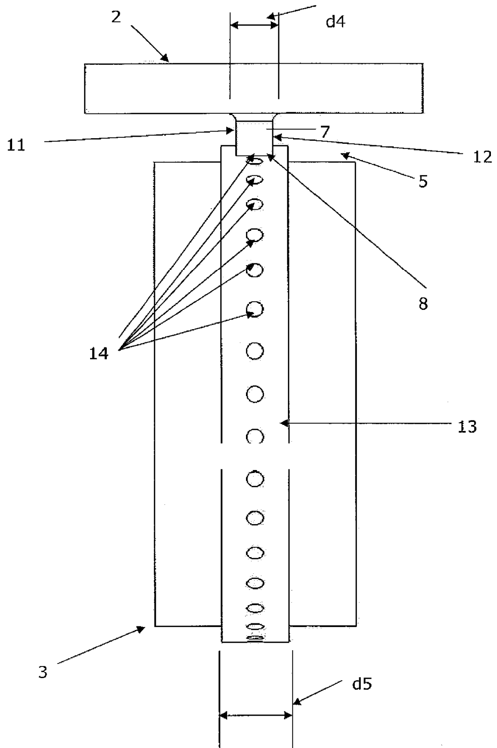
Figura 3: Alzado frontal de la escobilla y rueda con hoyuelos superficiales.
