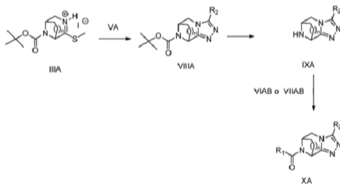
Esquema 3
