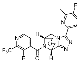
Ejemplo 162: (2,3-diclorofenilo)(6R,10S)-3-(5-fluoro-6-metilpiridina-2-ilo)-6,7,9,10-tetrahidro-5H-6,10-epimino[1,2,4]triazolo[3,4-d][1,5]oxazocina-11-ilo)metanona.
