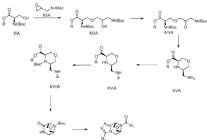
Esquema 4
