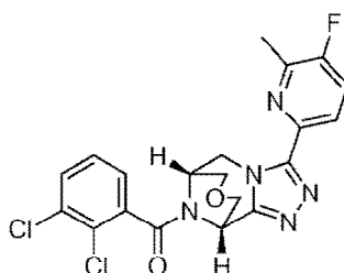
Ejemplo 163: (2-cloro-3-(trifluorometilo)fenilo)(6R,10S)-3-(4-(trifluorometilo)piridina-2-ilo)-6,7,9,10-tetrahidro-5H-6,10-epimino[1,2,4]triazolo[3,4-d][1,5]oxazocina-11-ilo)metanona.
