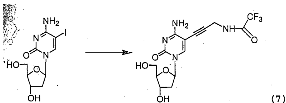
5-[3-(2,2,2-Trifluoroacetamido)-prop-1-ynil]-2'-desoxicitidina (7).
