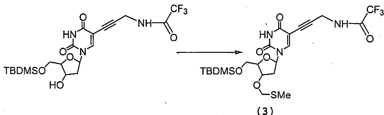
5'-O-(tert-Butidimetilsilil)-3'-O-metiltiometil-5-[3-(2,2,2-trifluoroacetamido)-prop-1-inil]-2'-desoxiuridina (3).
