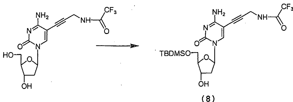
5'-O-(tert-Butyldimethylsilyl)-5-[3-(2,2,2-trifluoroacetamido)-prop-1-ynil]-2'-desoxycitidina (8).
