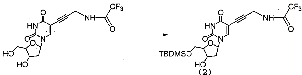
5'-O-(tert-butidimetilsilil)-5-[3-(2,2,2-trifluoroacetamido)-prop-1-inil]-2'-desoxiuridina (2).
